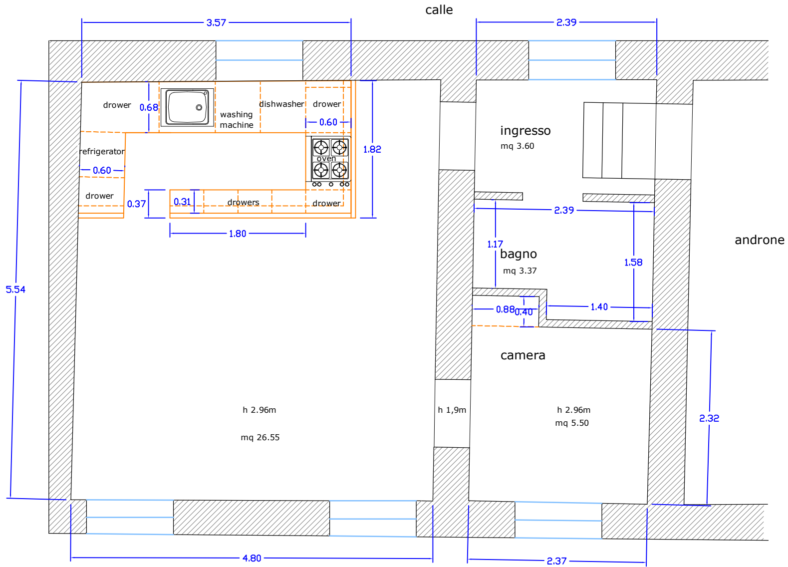
PIANTA APPARTAMENTO CA MOCENIGO
